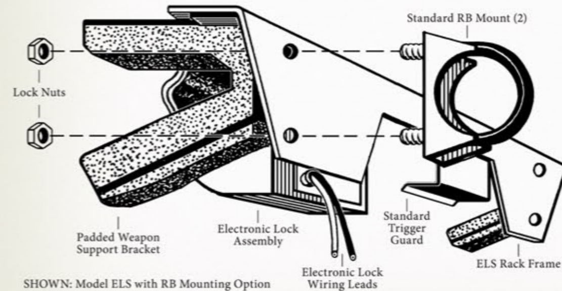
SHOWN: Model ELS with RB Mounting Option
